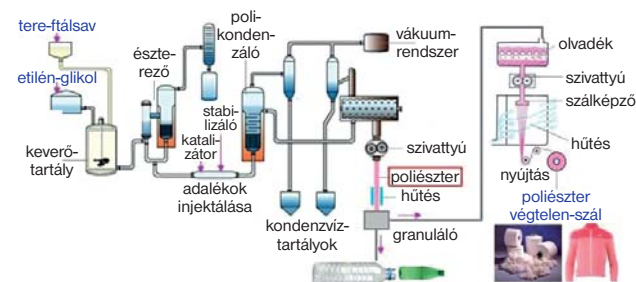
3. ábra. Az új előállítású poliészter képzése
