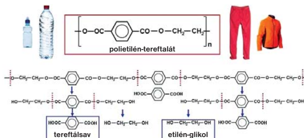
6. ábra. A PET depolimerizációja a kémiai újrahasonosítás során
