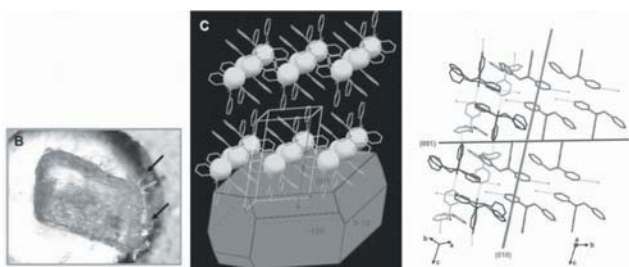
9. Ábra. A 4-(1-hidroxi-1,2-difeniletil)piridin HCl sójának szublimációja. A szublimátum, mely csak a szerves vegyületet tartalmazza, az anyakristály azon lapjaira válik ki, melyekkel parciális izostrukturális mutat.
