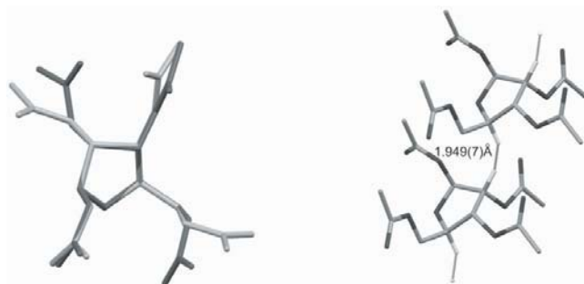
6. Ábra. Konformáció, intermolekuláris távolságok és kölcsönhatások, polimorfia: az 1,2,3,5-tetra-O-acetil- \beta -D-ribofuranóz módosulatai. A két módosulat konformációja. a.) A: instabil (világos szürke) monoklin , P2_1 ; B: stabil (sötét szürke) rombos , P2_12_1 . b.) A tasztító H...H intermolekuláris kölcsönhatás az instabil formában.
